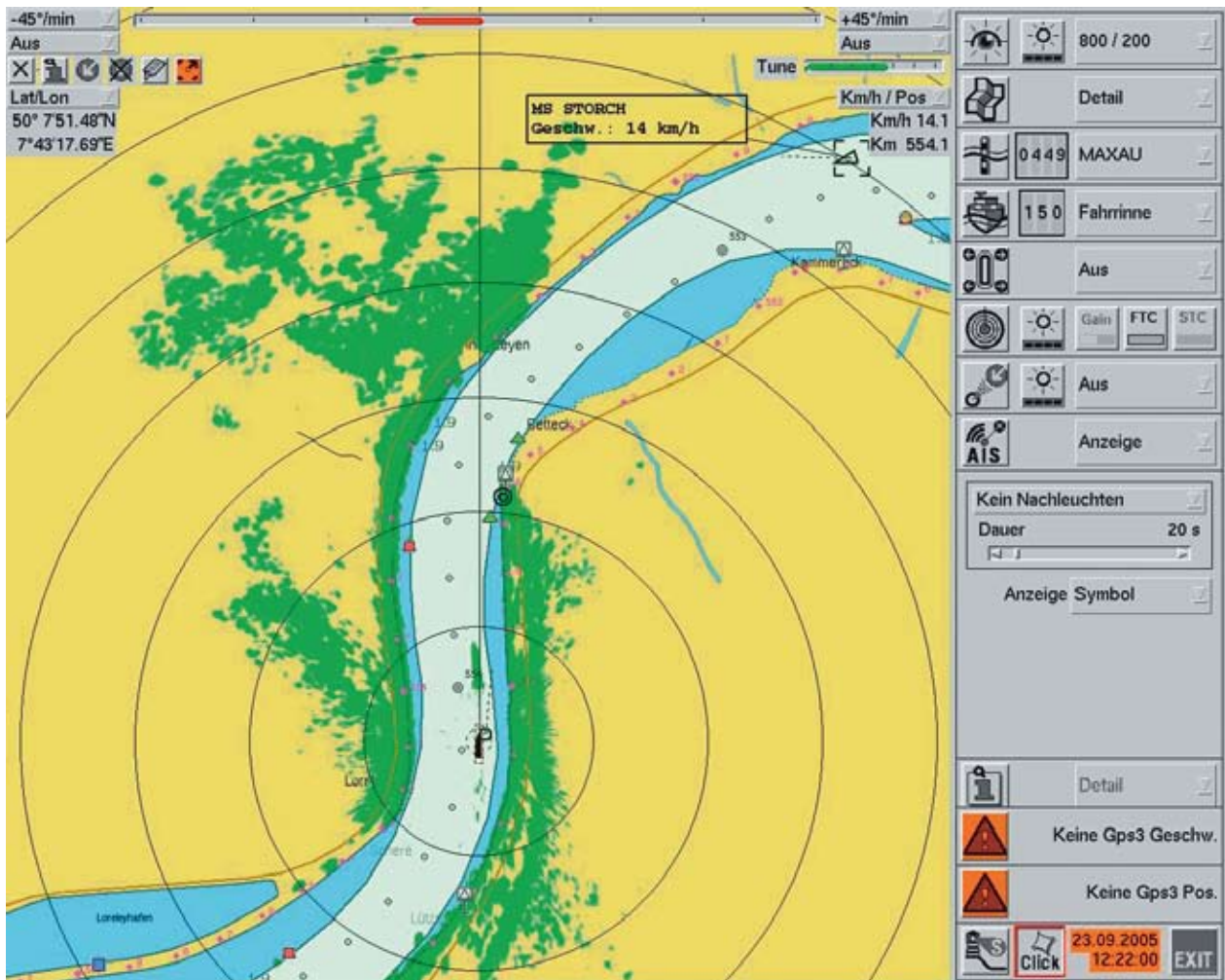
Inland ECDIS-System im Navigationsmodus
