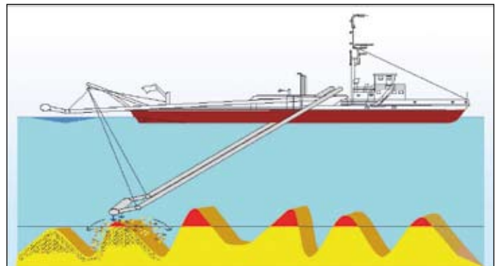
Skizze Wasserinjektionsgerät
