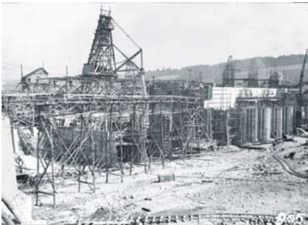
Bau der Anlage Kachlet ca. 1924
