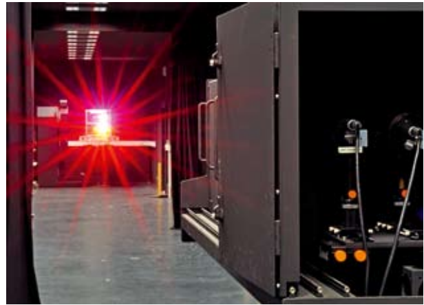
Blick ins Lichtlabor (Fotogoniometer)
