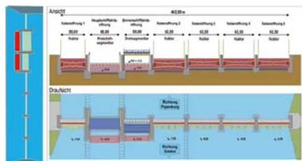
Variante: Zwei Drehsegmente als Sohlschwelle und vorhandene Hubtore (Grafik: IMS)
